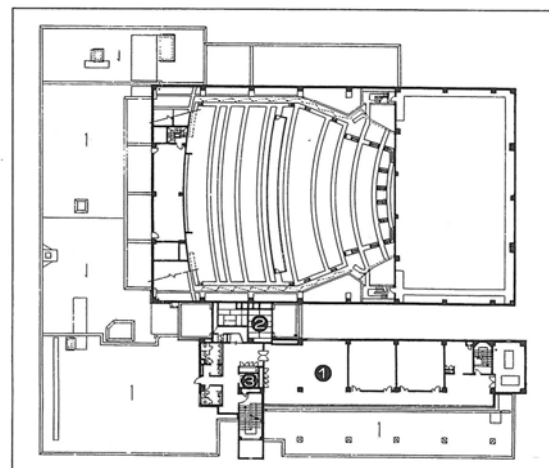
4階平面図
