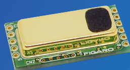
CDM7162 NDIR 式 CO 2 ガスセンサ
